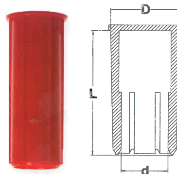
Obr. 2 – Rychlá krytka GAQ a její řez
